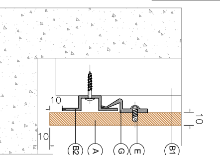
Escala / Scale: 1/3
