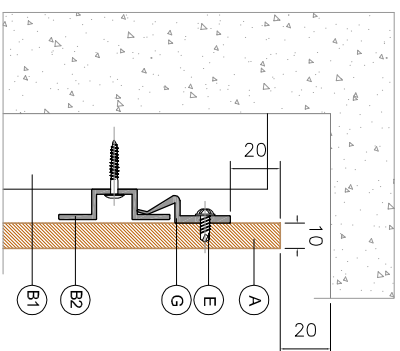
Escala / Scale: 1/3
