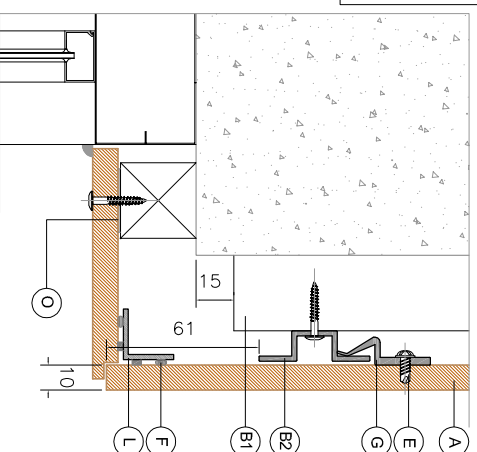
Escala / Scale: 1/3
