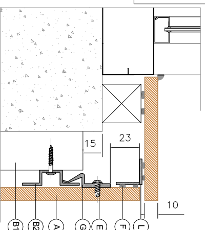
Escala / Scale: 1/3
