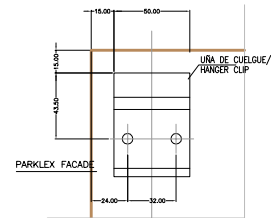
URSA EN ESQUINA SUPERIOR/ HANGER CLIP ON TOP EDGE
