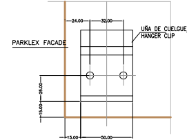
URSA EN ESQUINA INFERIOR/ HANGER CLIP ON BOTTOM EDGE
