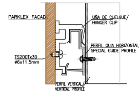
URSA SOBRE PERFIL/ HANGER CLIP OVER PROFILE
