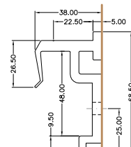
URSA DE CUELQUE/ HANGER CLIP
